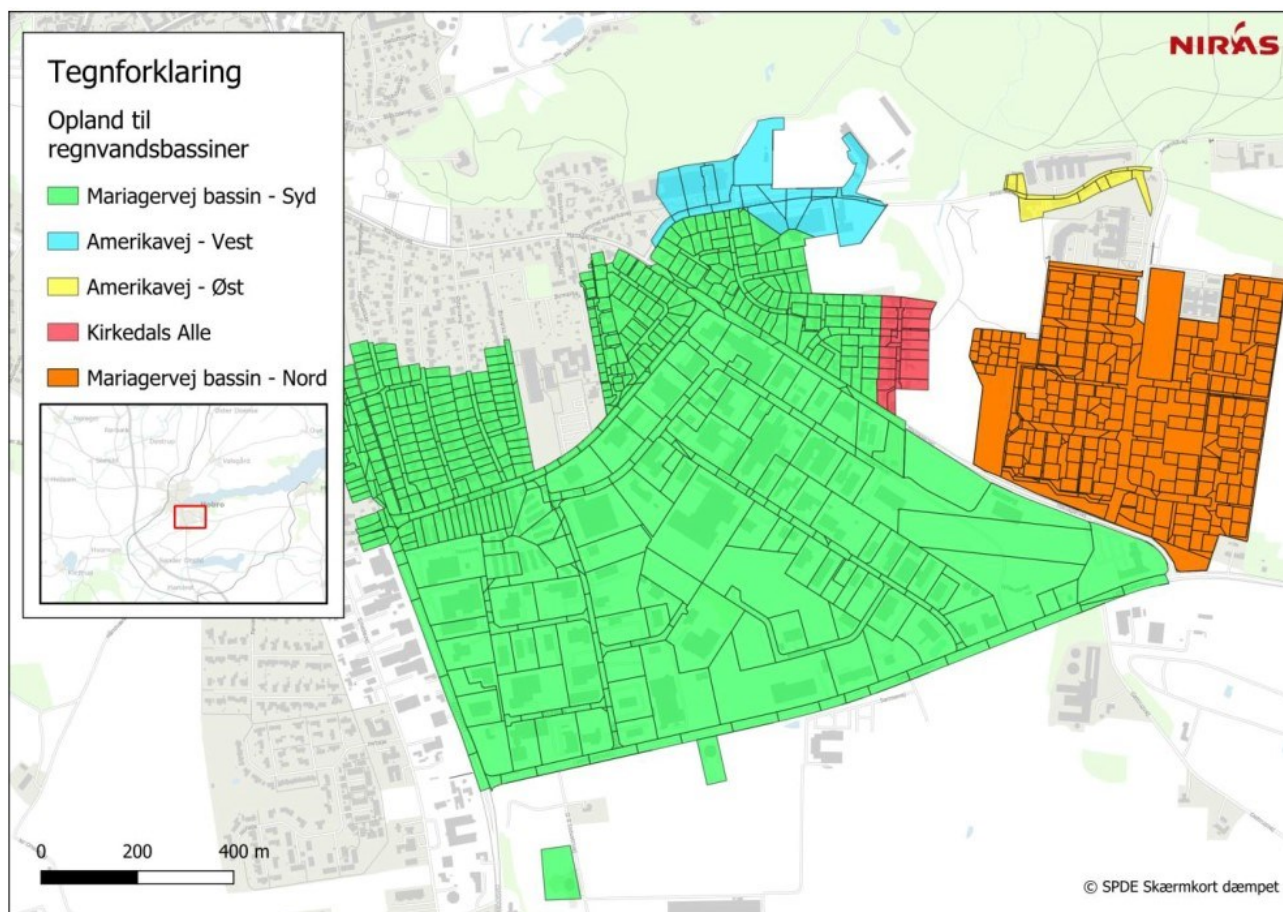
Figur 3.1: Oplande med planlagt udløb til Kirkedalsbækken.
